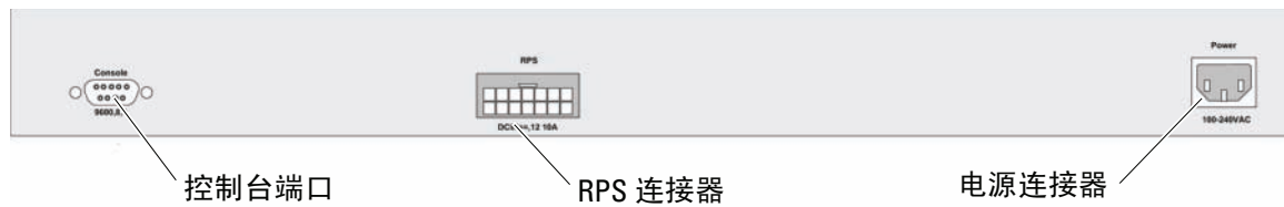
PowerConnect 3524/3548 后视图
