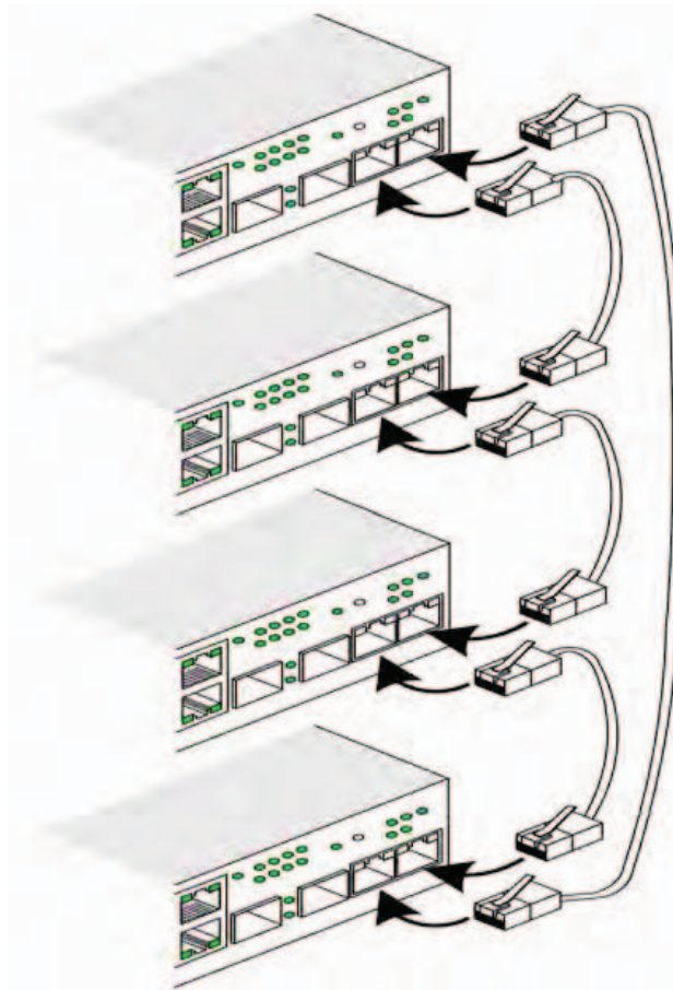
Abbildung 2-1. Stacking-Verkabelungsschema
